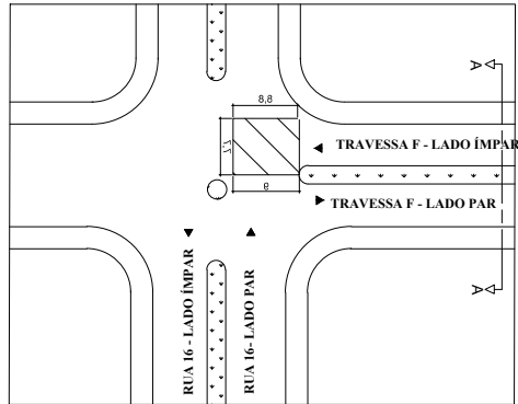
01. PLANTA DE SITUAÇÃO ESC: 1/1000
