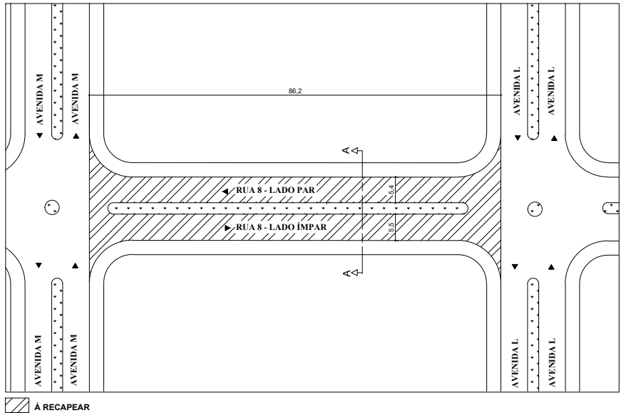
01.PLANTA DE SITUAÇÃO ESC: 1/1000
