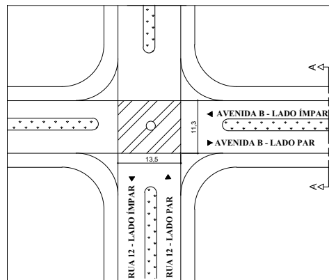
01. PLANTA DE SITUAÇÃO ESC: 1/1000
