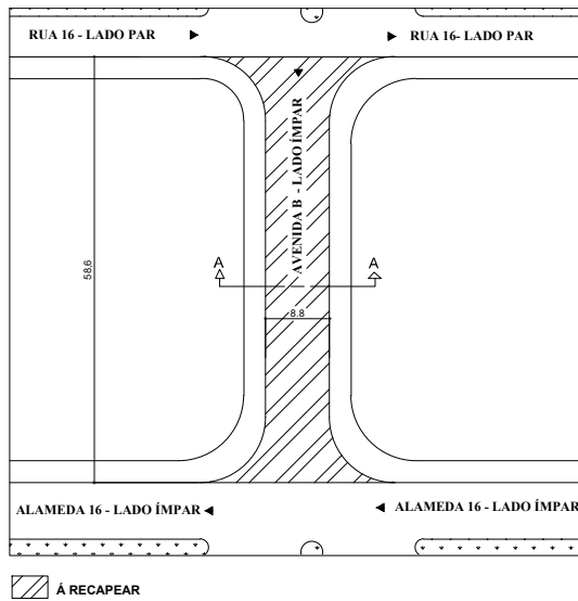
01. PLANTA DE SITUAÇÃO ESC: 1/1000
