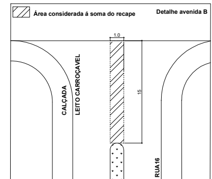
04. DETALHE DA EXTREMIDADE DO CANTEIRO
