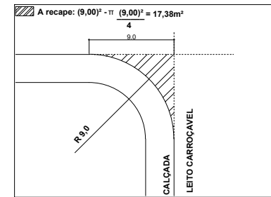
05. DETALHE DA EXTREMIDADE DO CANTEIRO
