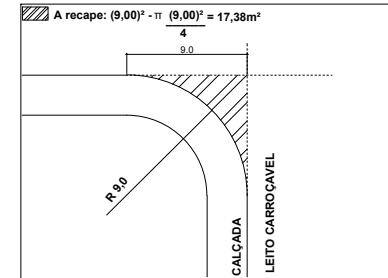
03. DETALHE DO RAIO ESC: 1/10
