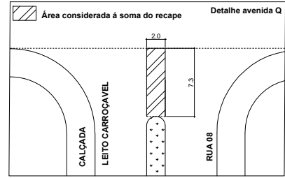
04. DETALHE DA EXTREMIDADE DO CANTEIRO ESC: 1/50
