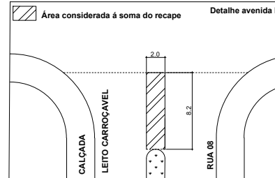
03. DETALHE DA EXTREMIDADE DO CANTEIRO ESC: 1/50
