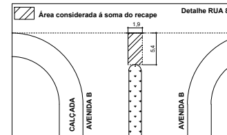
06. DETALHE DA EXTREMIDADE DO CANTEIRO ESC: 1/50
