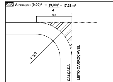
03. DETALHE DO RAI ESC: 1/10
