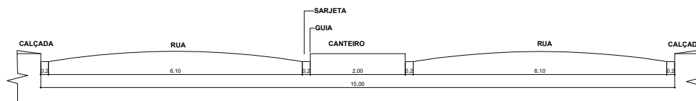
02. CORTE TRANSVERSAL A-A DAS RUAS ESC: 1/100
