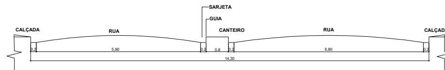
02. CORTE TRANSVERSAL A-A DAS RUAS ESC: 1/100
