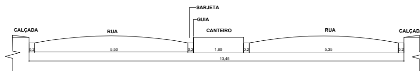
02. CORTE TRANSVERSAL A-A DAS RUAS ESC: 1/100
