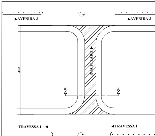
01. PLANTA DE SITUAÇÃO ESC: 1/1000
