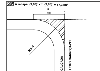
04. DETALHE DO RAIO ESC: 1/10
