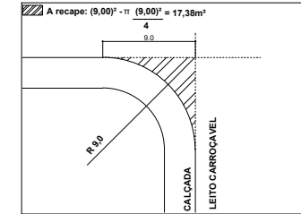
05. DETALHE DA EXTREMIDADE DO CANTEIRO ESC: 1/50
