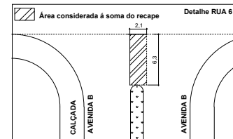
06. DETALHE DA EXTREMIDADE DO CANTEIRO
