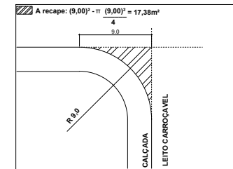
05. DETALHE DA EXTREMIDADE DO CANTEIRO
