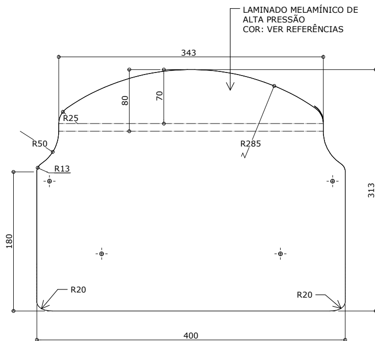
VISTA SUPERIOR
