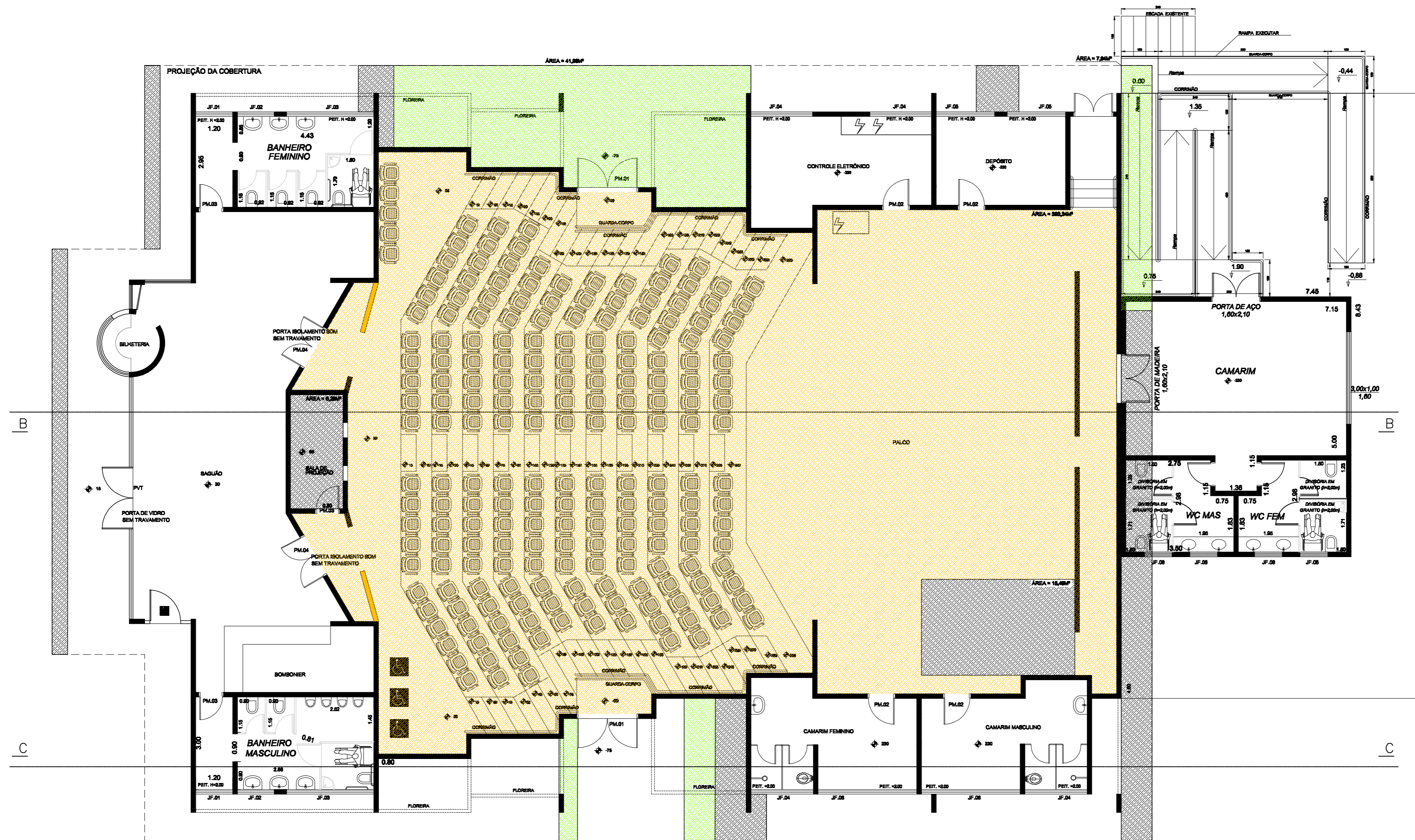
PLANTA - TEATRO ESCALA 1:100
