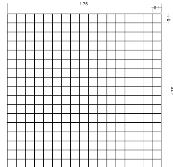
04 - DETALHE DA ARMAÇÃO NA TAMPA SUPERIOR
