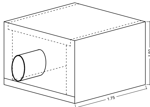
05 - DIMENSÕES DA CAIXA
