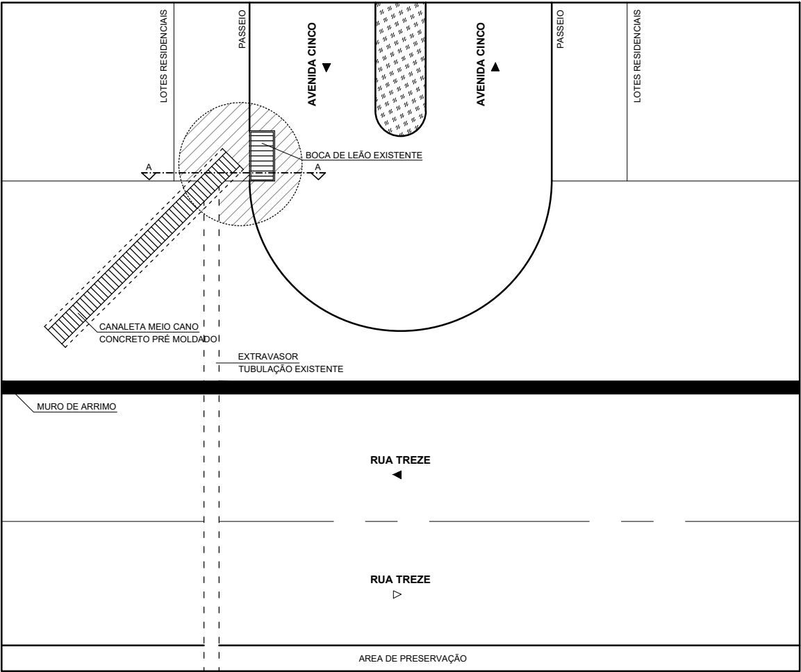
01 - PLANTA DE SITUAÇÃO ESC: 1/200
