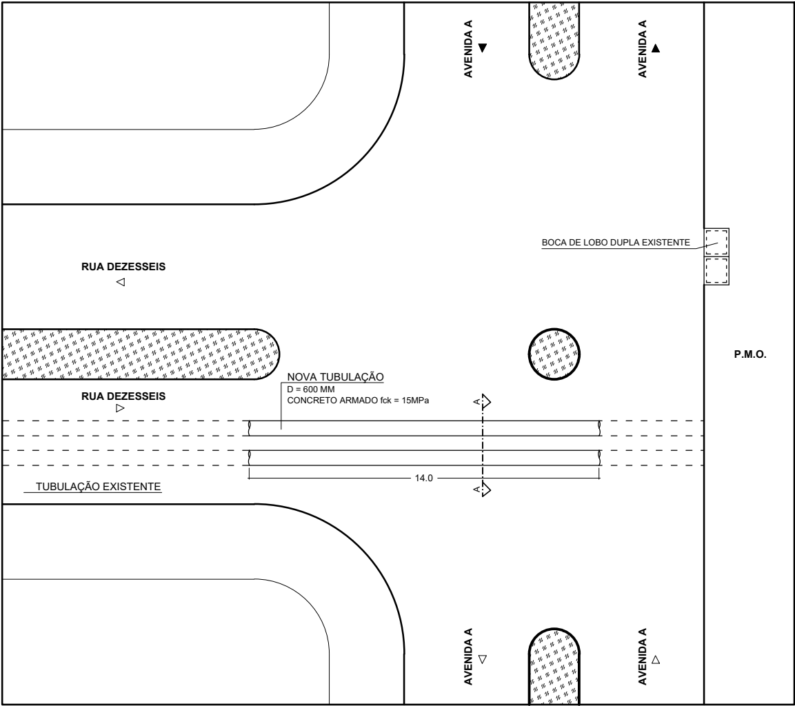
01 - PLANTA DE SITUAÇÃO ESC: 1/200
