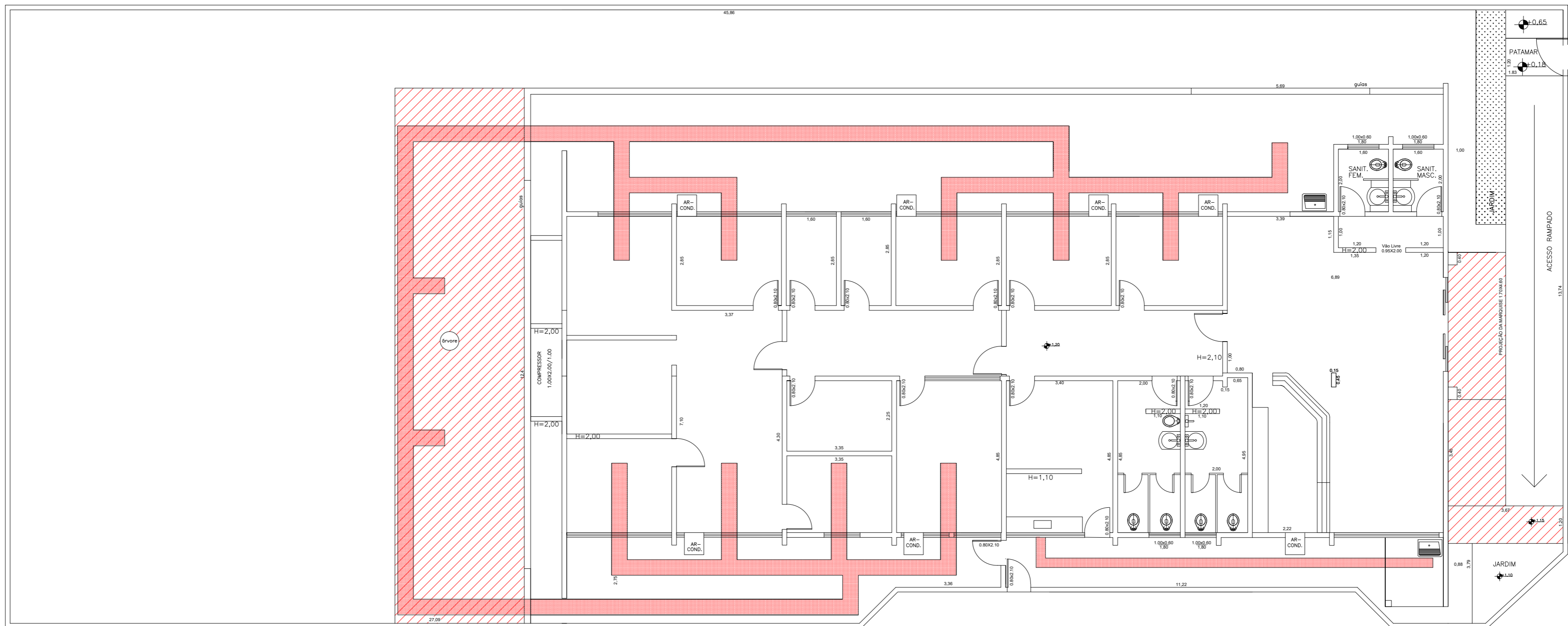
Planta Baixa - Preparo do Terreno Escala 1:100
