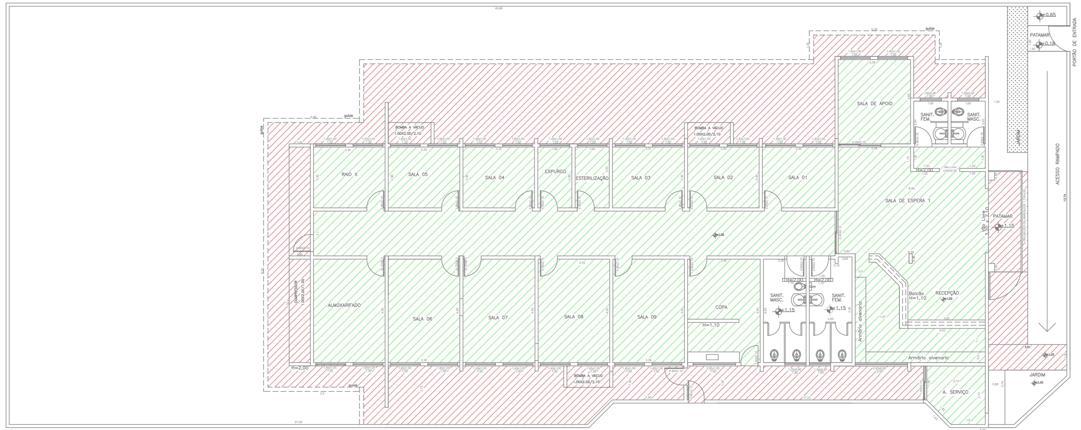
Planta Baixa - Piso Escala 1:100
