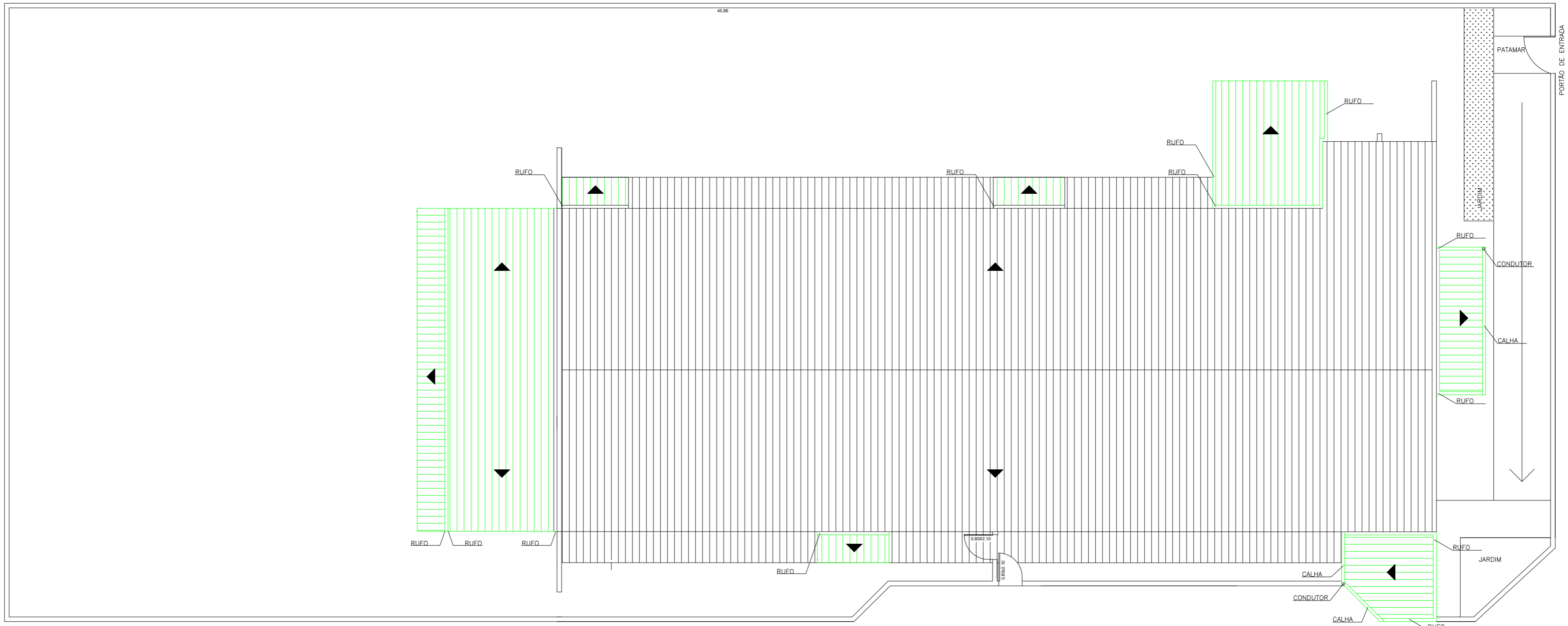
Planta Baixa - Cobertura Escala 1:100
