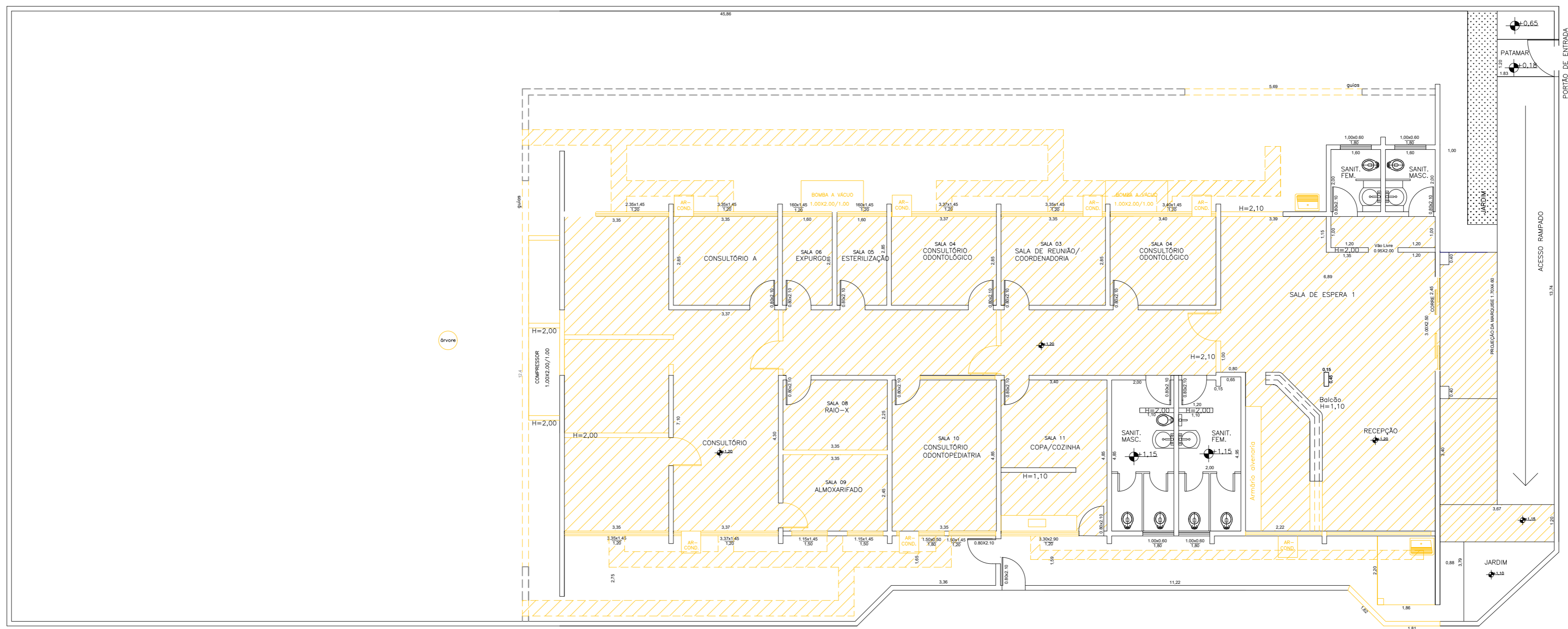
Planta Baixa - Demolições e Retiradas Escala 1:100
