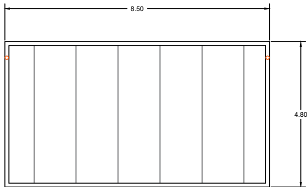
PLANTA BAIXA ESC 1/100 COBERTURA DE POLICARBONATO EM CURVA COM CALHA E PÉ DIREITO 8,50 X 4,80
