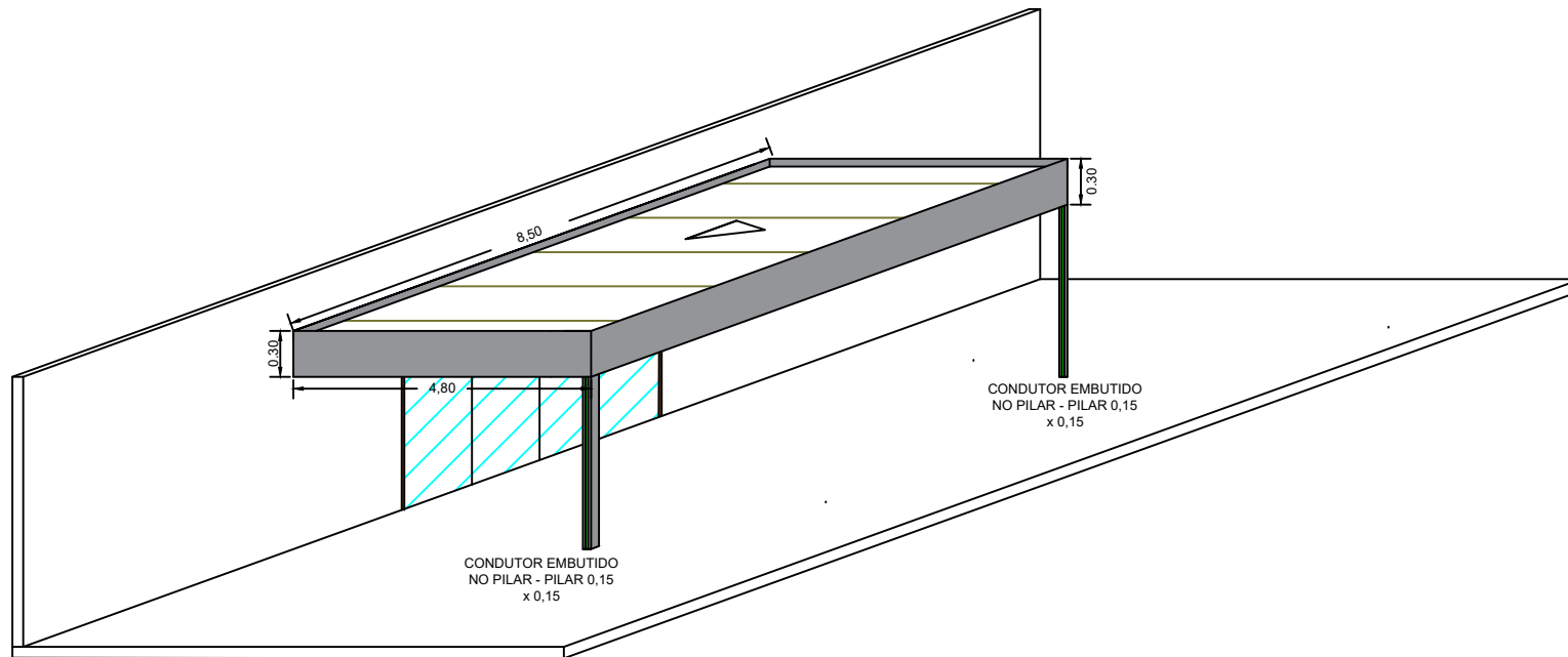
PERSPECTIVA ESC 1/100
