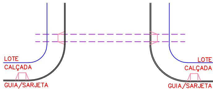
VISTA SUPERIOR - RAMPAS EM PASSEIOS SEM ESCALA
