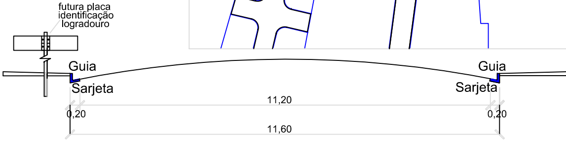
SEÇÃO TRANSVERSAL A-A DAS RUAS (Leito Carroçável de 11,60m) ESCALA. 1:200
