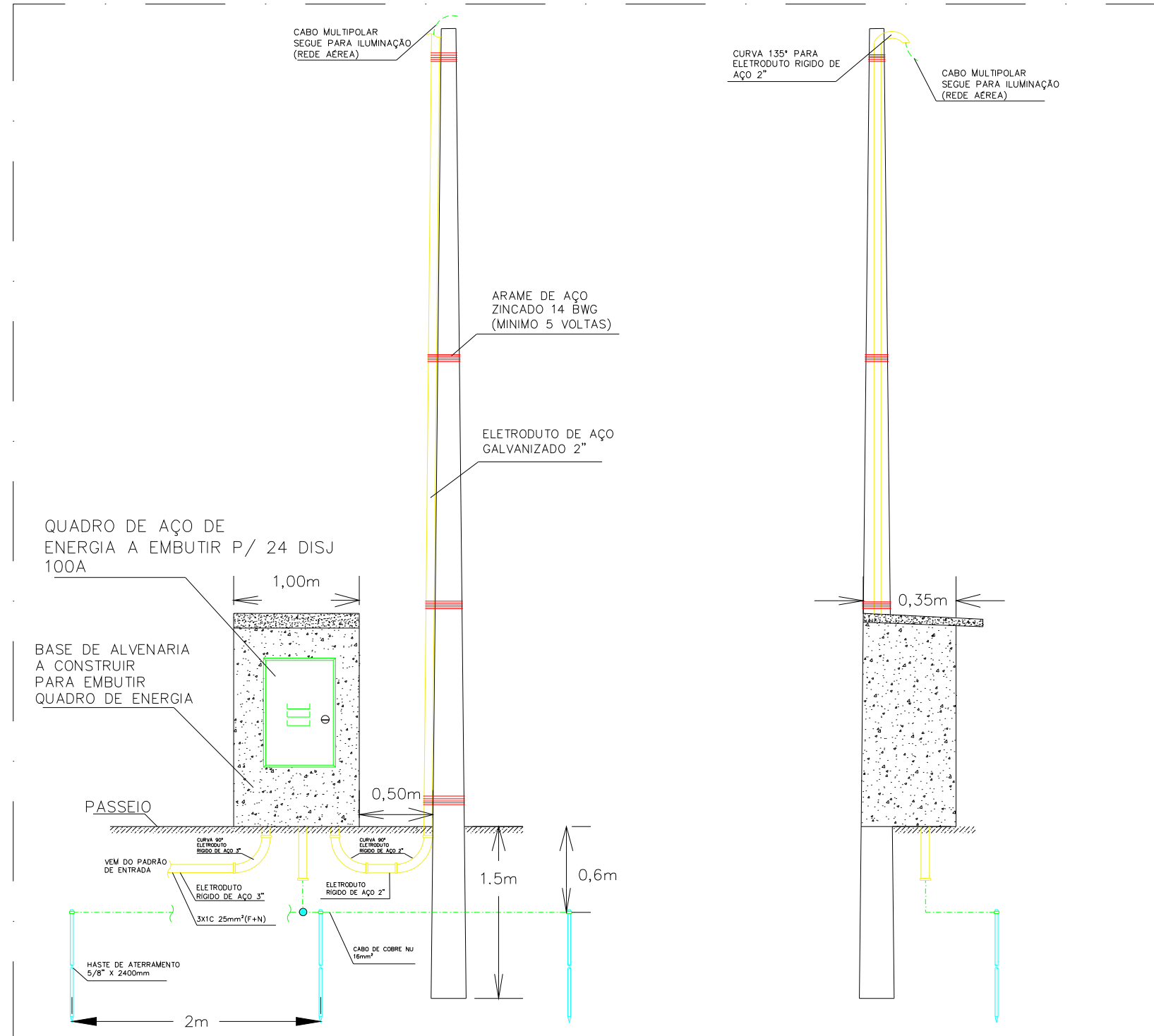
DETALHE 01 – LIGAÇÃO QUADRO DE ENERGIA PARA O POSTE DE REDE AÉREA S/ ESCALA
