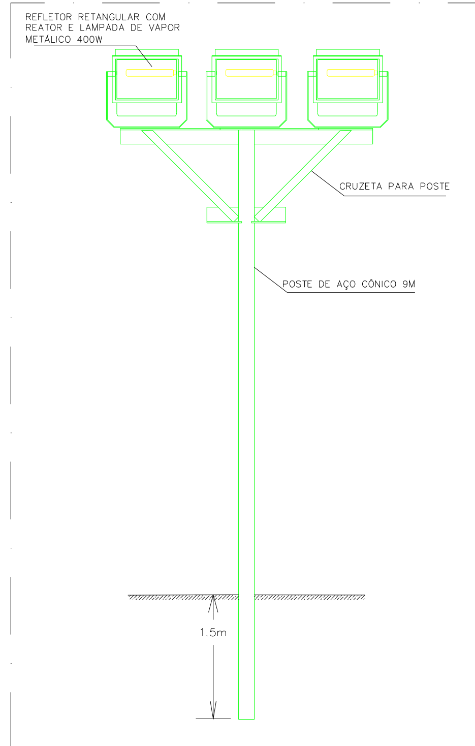
DETALHE 02 – INSTALAÇÃO DOS REFLETORES NO POSTE S/ ESCALA
