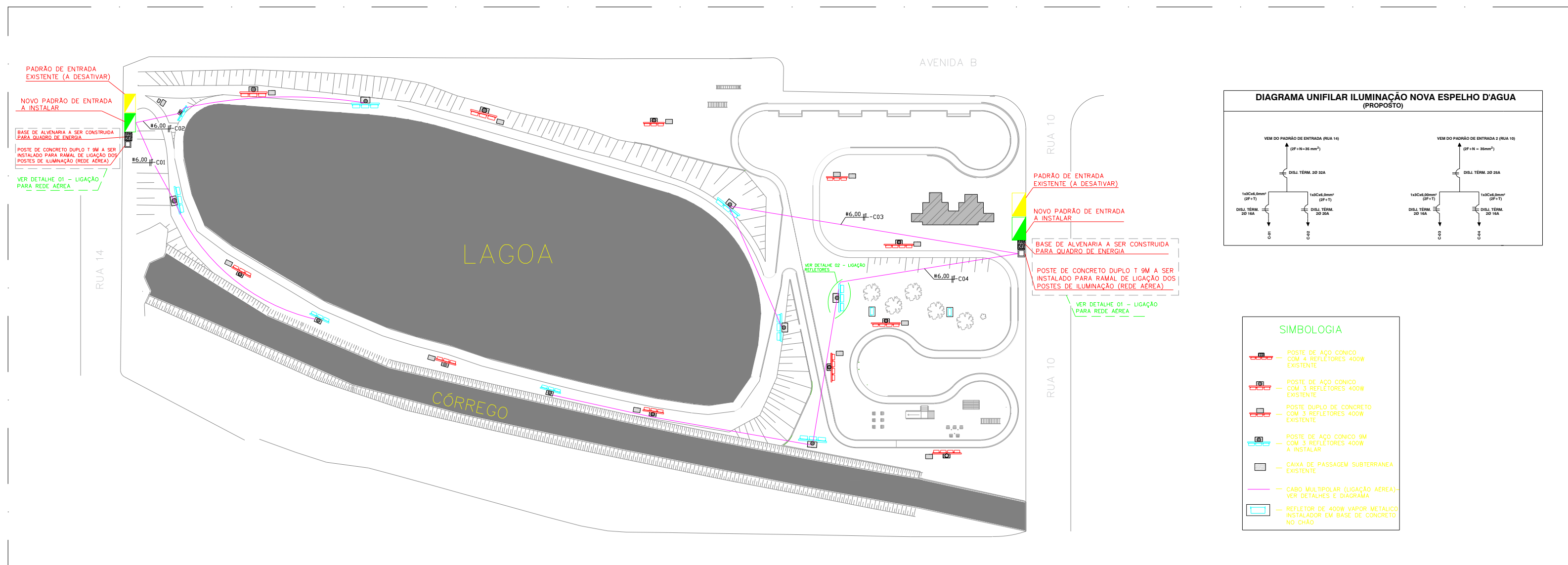
PLANTA BAIXA DE LIGAÇÃO DA REFORMA DA ILUMINAÇÃO E PADRÕES DE ENTRADA ESCALA 1:100
