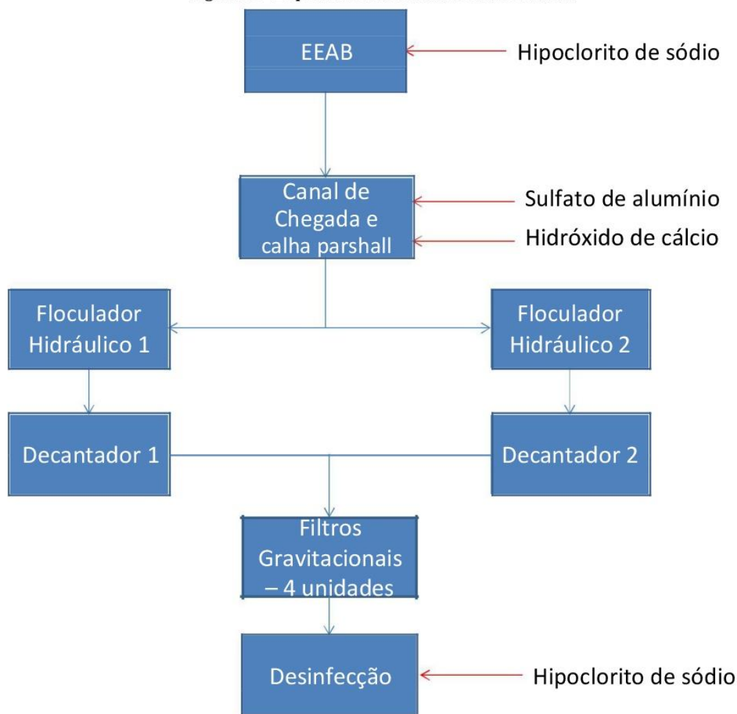
Figura 18 – Esquema de funcionamento ETA Orândia
