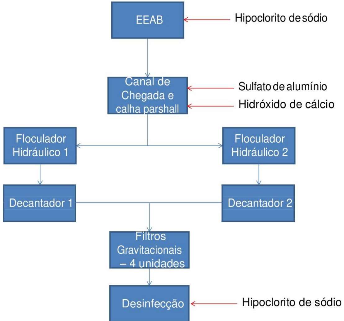
Figura 18 – Esquema de funcionamento ETA Orlandia
