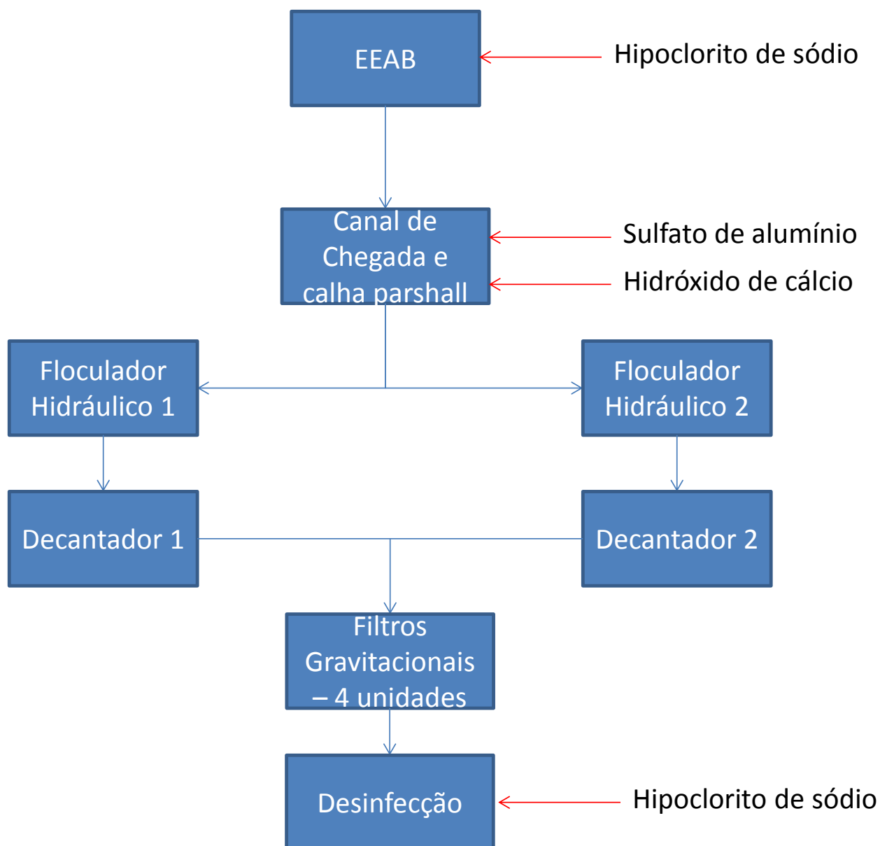
Figura 18 – Esquema de funcionamento ETA Orlândia
