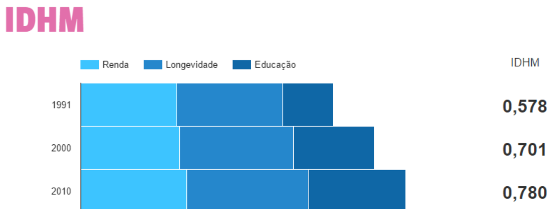
Figura 2 – Composição do IDHM do município de Orlândia
