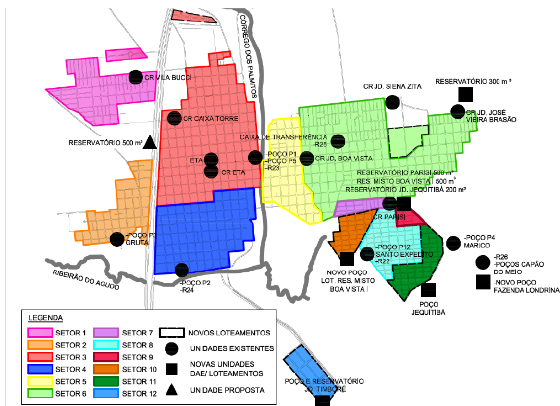
Figura 64 – Setorização proposta para Orlândia
